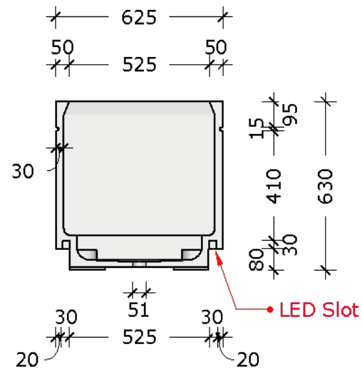
4 Section View Scale: 1 : 20
