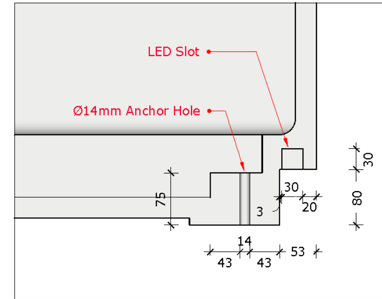
2 Zoomed View A Scale: 1 : 5 @A3
