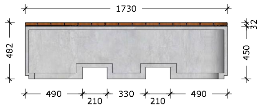
4 Longitudinal Section
