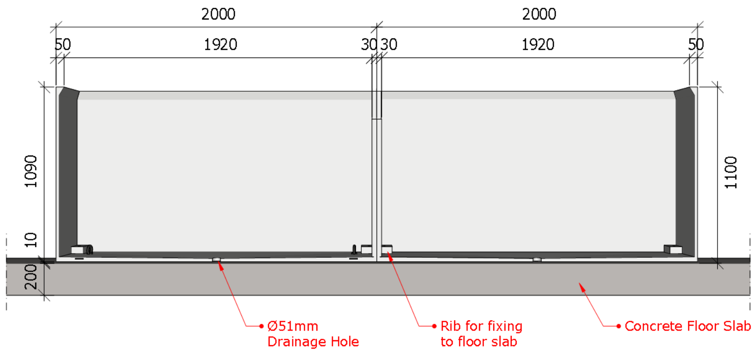
Longitudinal Section
